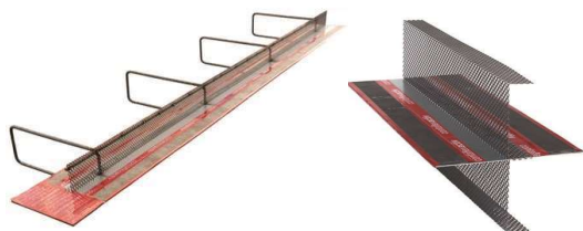
Avstängare Bentonit nr 8 (2,25 m/st) Produceras projektanpassad i efterfrågad höjd och med byglar för förenklat montage Avstängare Bentonit nr 18 (2,25 m/st) Utan byglar. Finns lagerlagd
