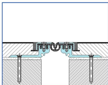
Bild 3: Eftermonterad
