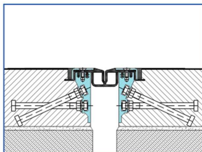
Bild 4: Förmonterad
