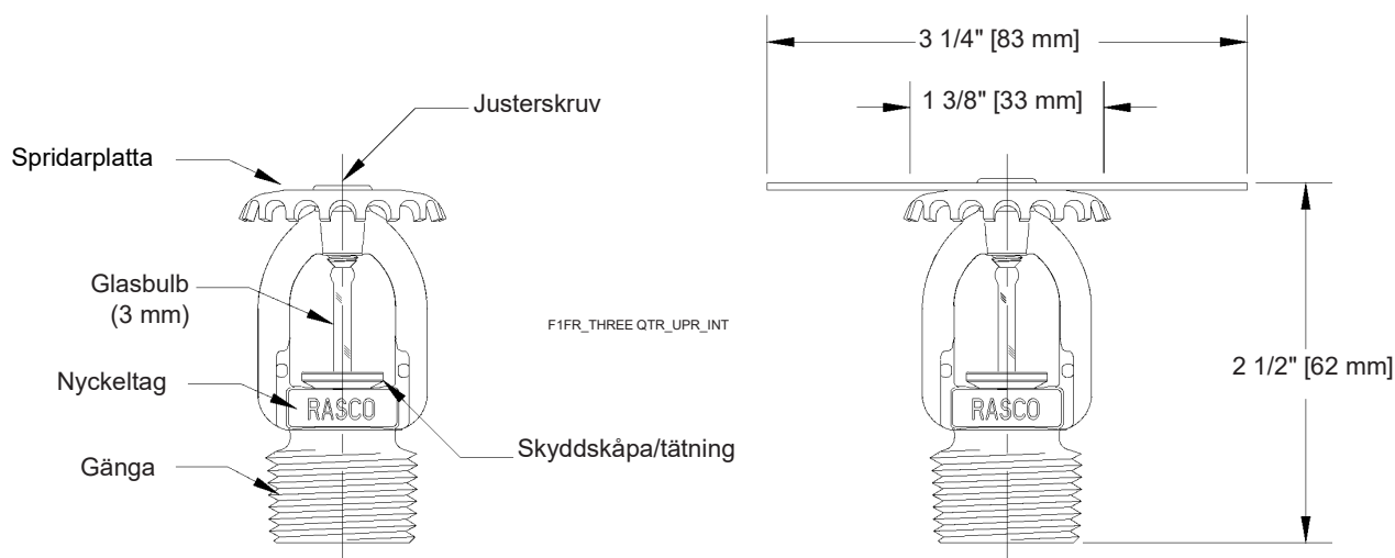
Uppåtriktad sprinkler modell F1FR80, komponenter och mått
