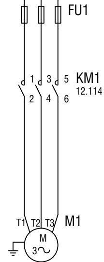
COMPRESSOR 1 KOMPRESSOR 1
