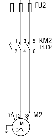
COMPRESSOR 2 KOMPRESSOR 2
